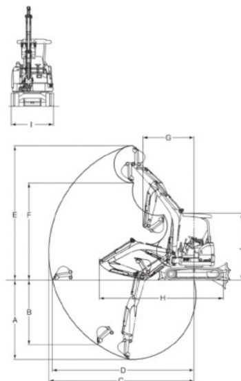
外形図及び作業範囲図
