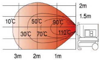
●温度分布図(上昇温度0℃基準)
