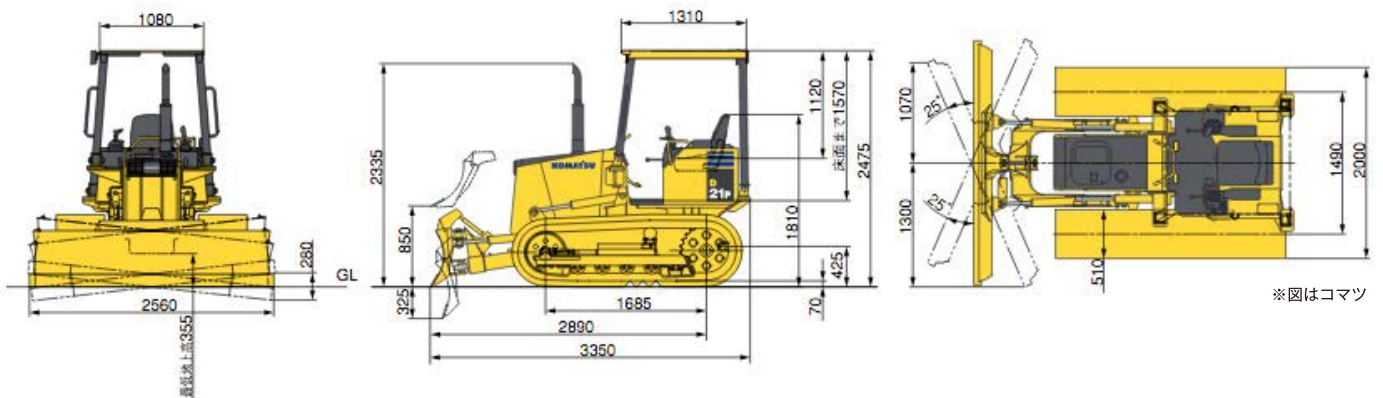
外形図及び 作業範囲図
