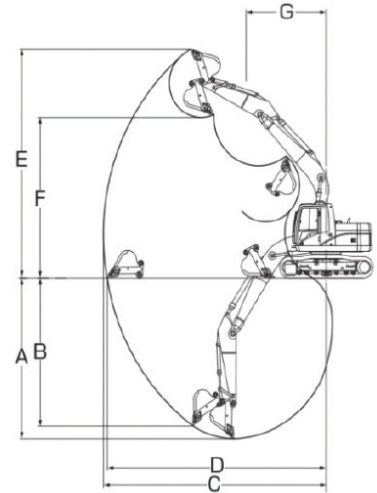
外形図及び 作業範囲図
