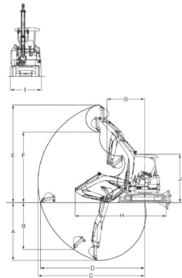
外形図及び 作業範囲図
